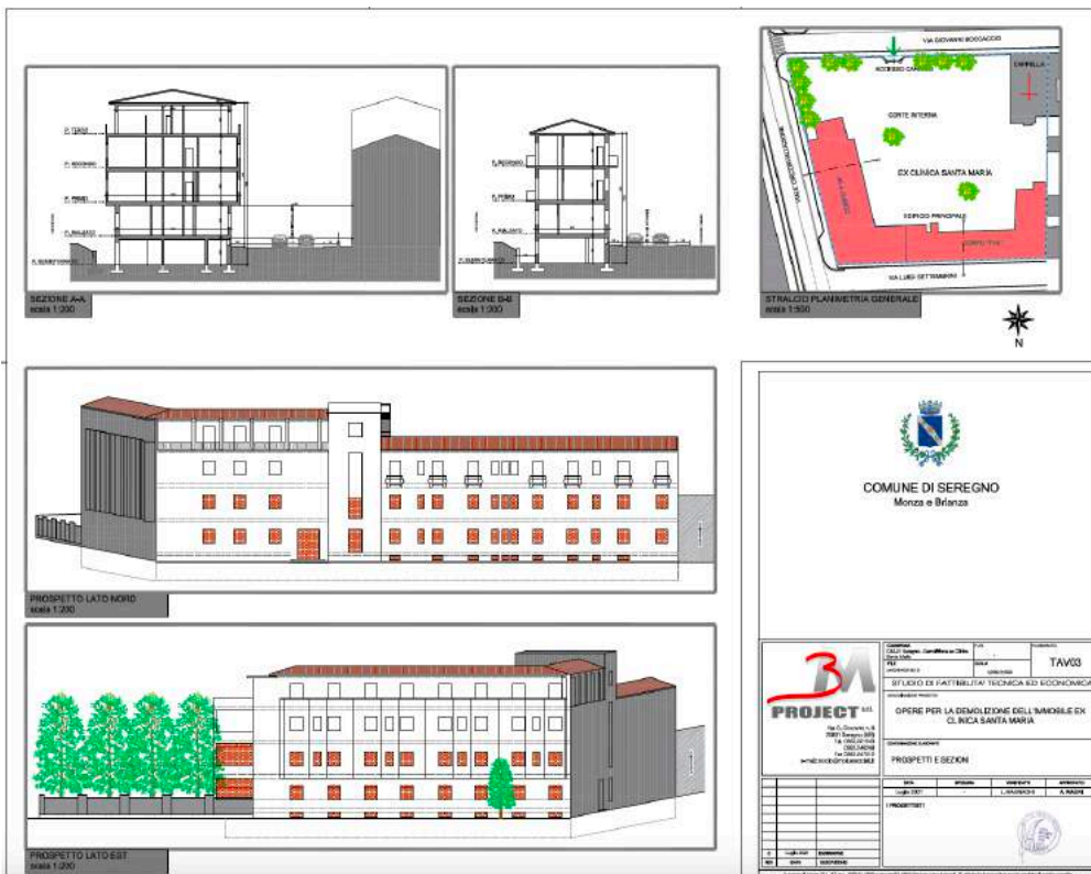
Prospetti e sezioni dei corpi di fabbrica demoliti
